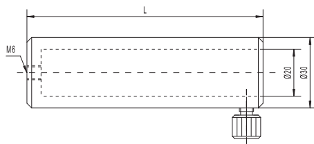
尺寸图:
